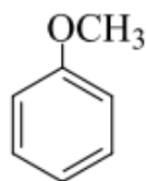
Anisole
