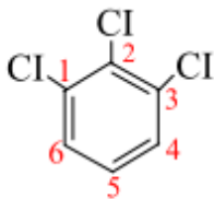
1,2,3-trichlorobenzene
