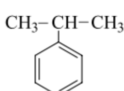
Cumene
