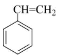
Styrene
