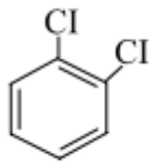
O-dichlorobenzene
